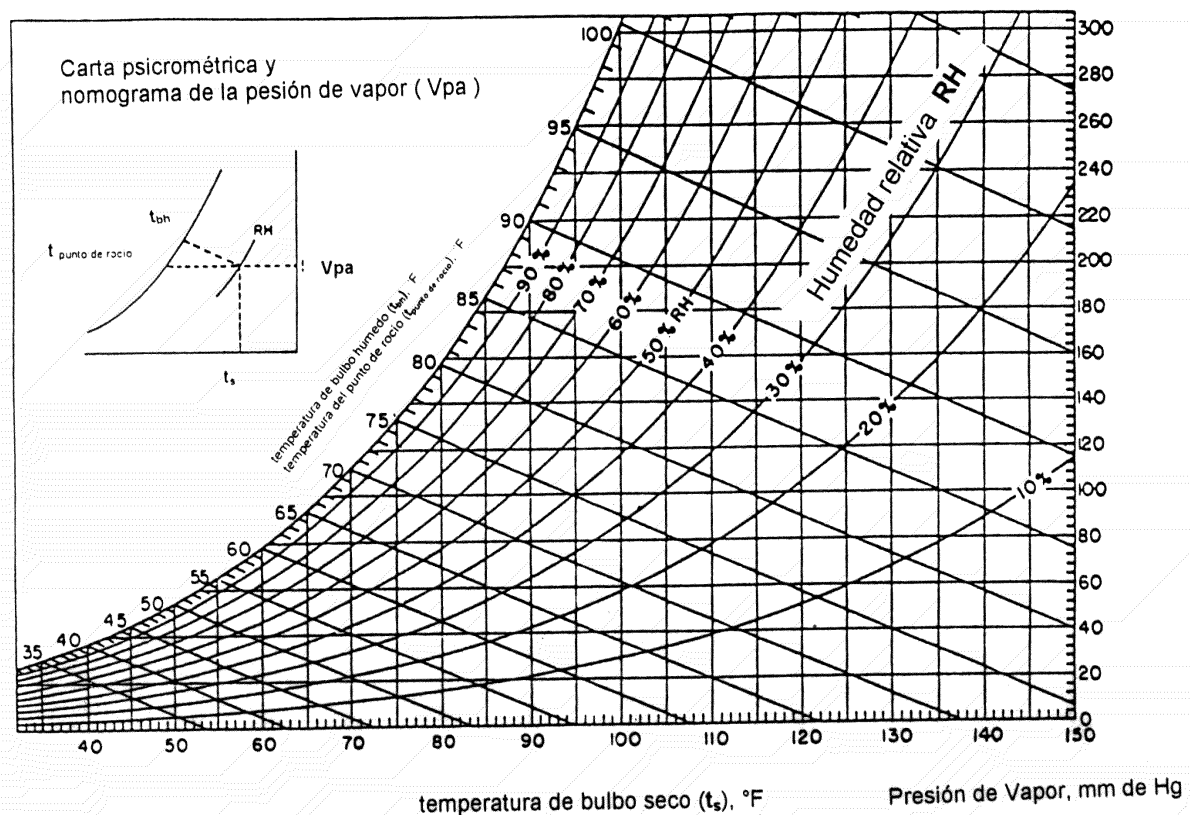
Carta psicrométrica
