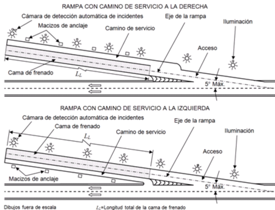
Figura 1.- Rampa de emergencia para frenado. Esquema de disposición en planta
