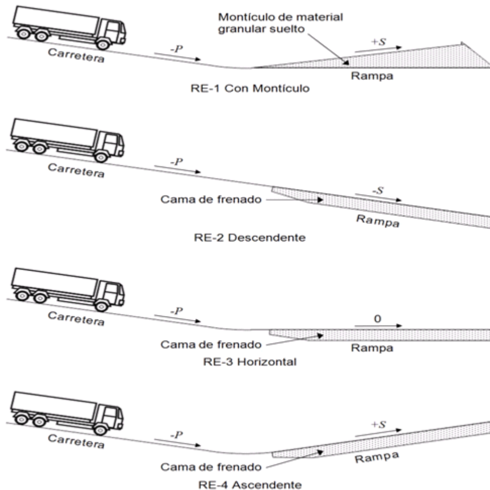
Figura 2.- Tipos de rampas de emergencia para frenado (RE)
