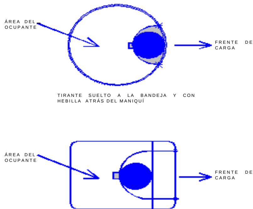
FIG. 3 TIRANTE ALREDEDOR DEL INFANTE SOBRE EL TUBO FRONTAL Y CHAROLA ALREDEDOR DEL MANIQUI CON UNA HEBILLA
