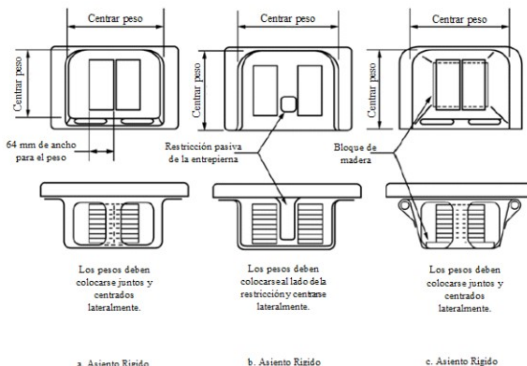
Figura 1-Arreglo de pesos para prueba de estabilidad
