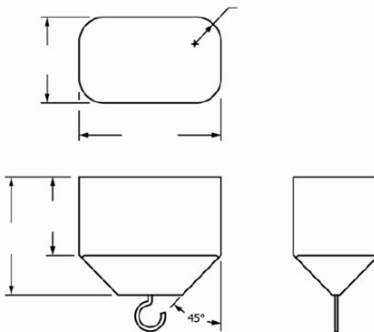
Figura 4-Bloque de cuña
