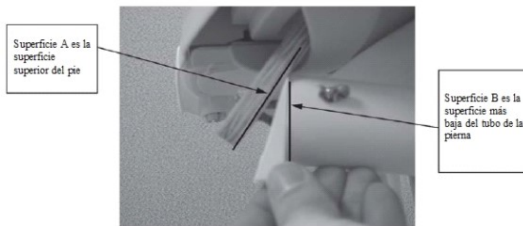
Figura 6-Bloque de 30°
