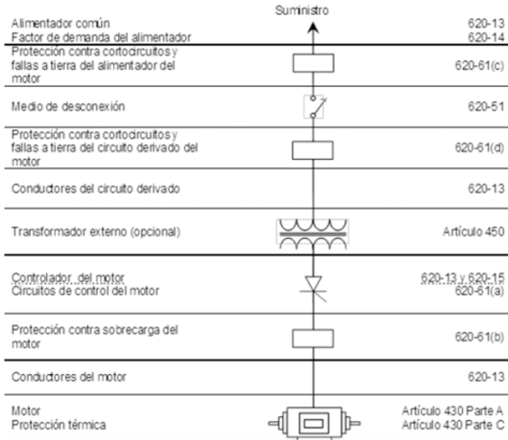
Figura 620-13.- Diagrama unifilar
