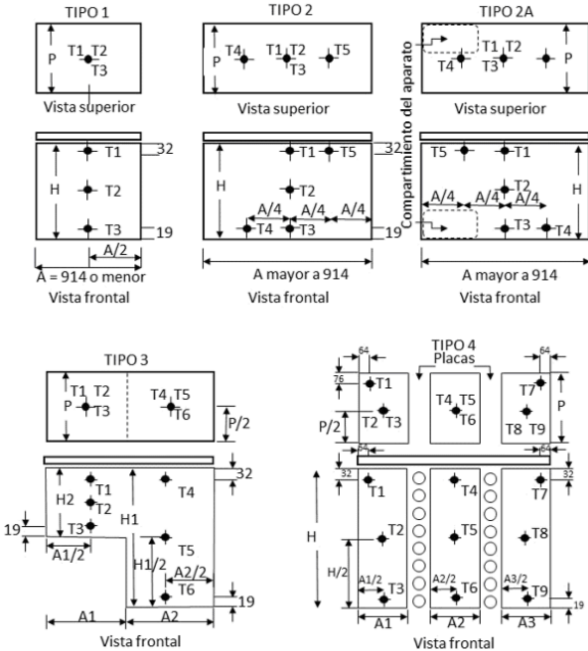
Figura A.3-Ubicación de los termopares para determinar las temperaturas de los compartimentos de alimentos frescos.
