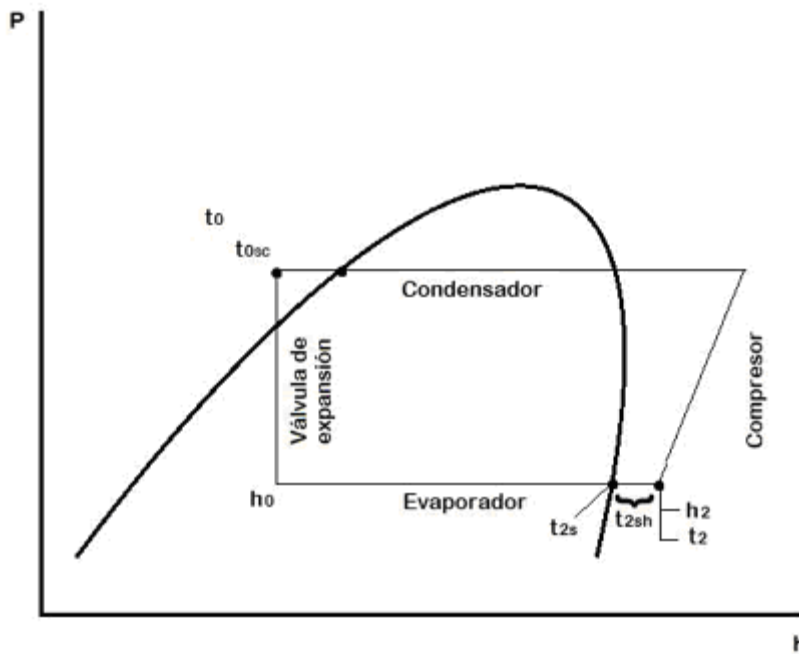
Figura 1. Diagrama presión vs entalpia con ciclo de refrigeración convencional.
