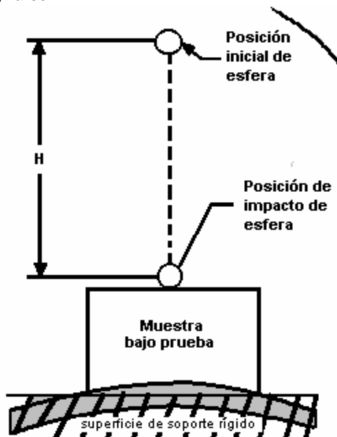
FIGURA 6.- Prueba de impacto usando una esfera
