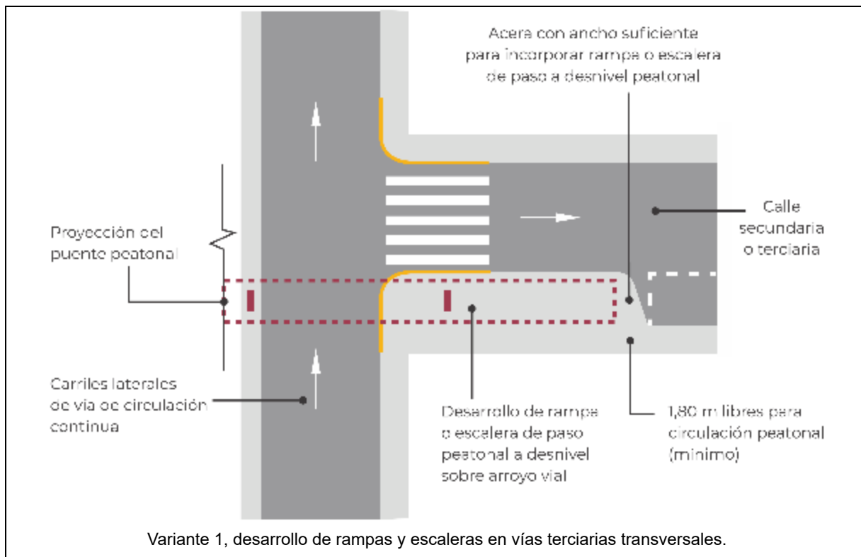
Figura 47.- Desarrollo de rampas y escaleras en pasos peatonales a desnivel para vías de circulación continua en aceras estrechas [1] [2]
