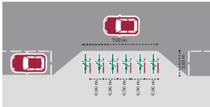
Variante 3, sobre carriles laterales o extensiones de acera en posición perpendicular.
