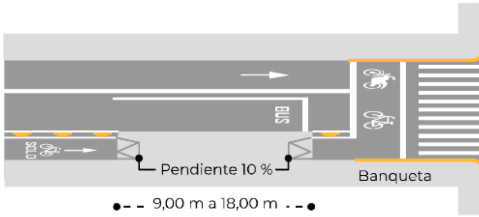
Variante 1, parada con plataforma a nivel de acera en cicloavía.
