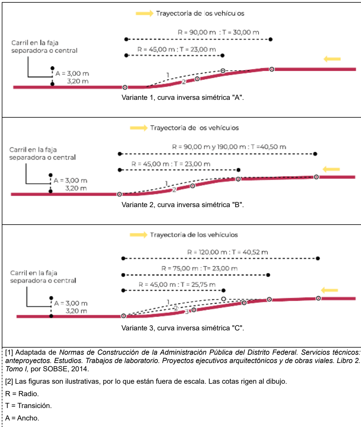
Figura 84.- Diseños de carril en la faja separadora central con remate en forma de punta de bala [1] [2]
