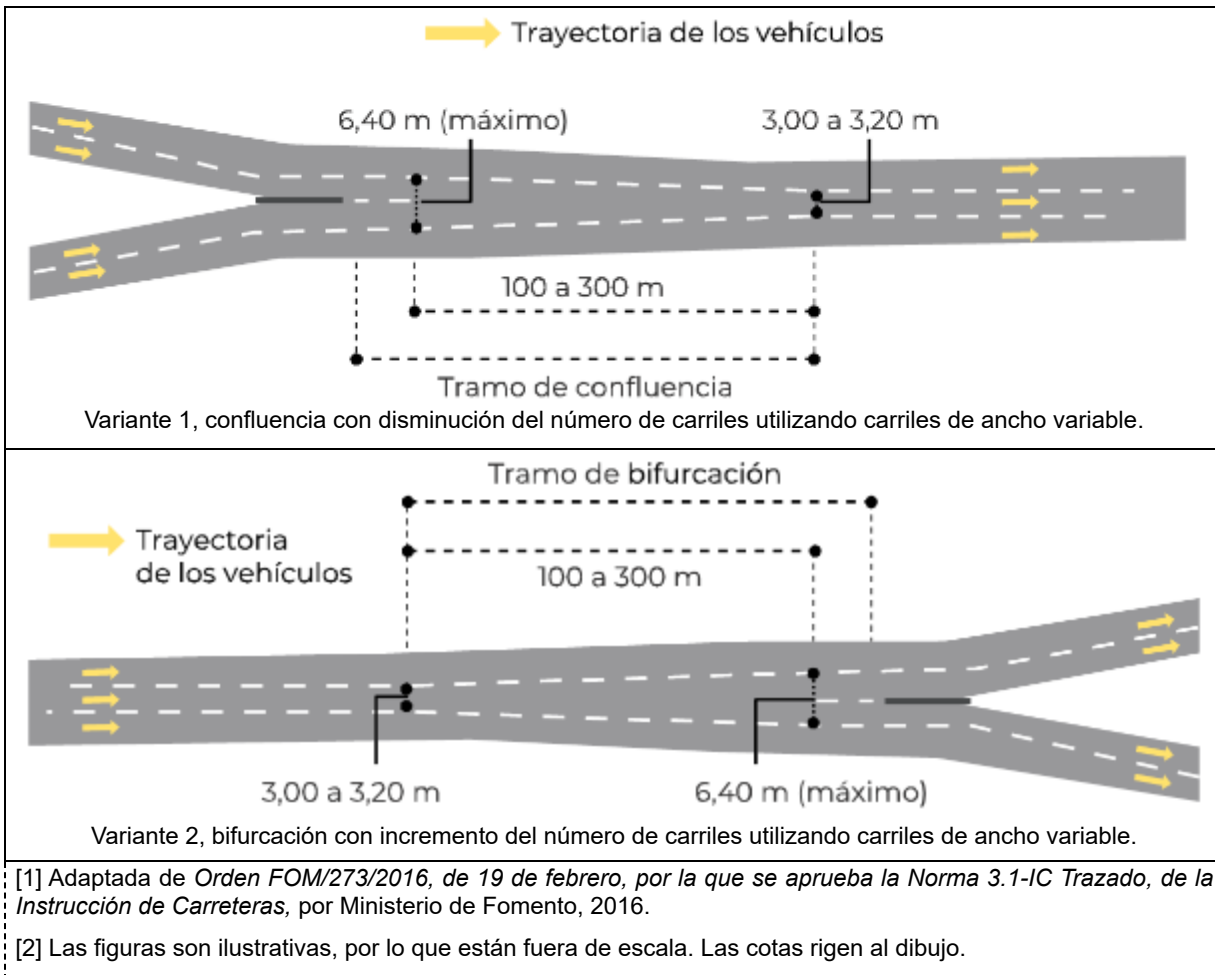
Figura 26.- Modificación de número de carriles con ancho variable [1] [2]
