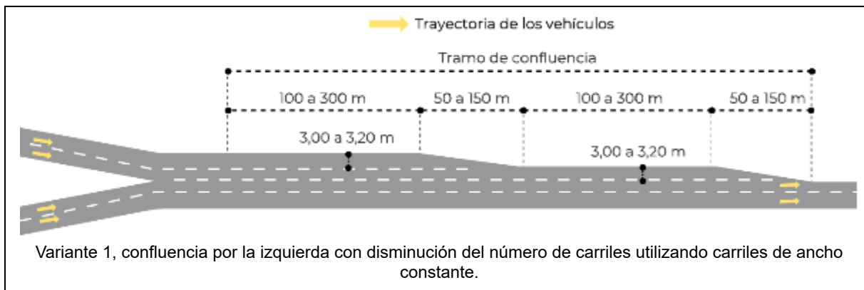
Figura 25.- Transiciones con modificación en el número de carriles [1] [2]
