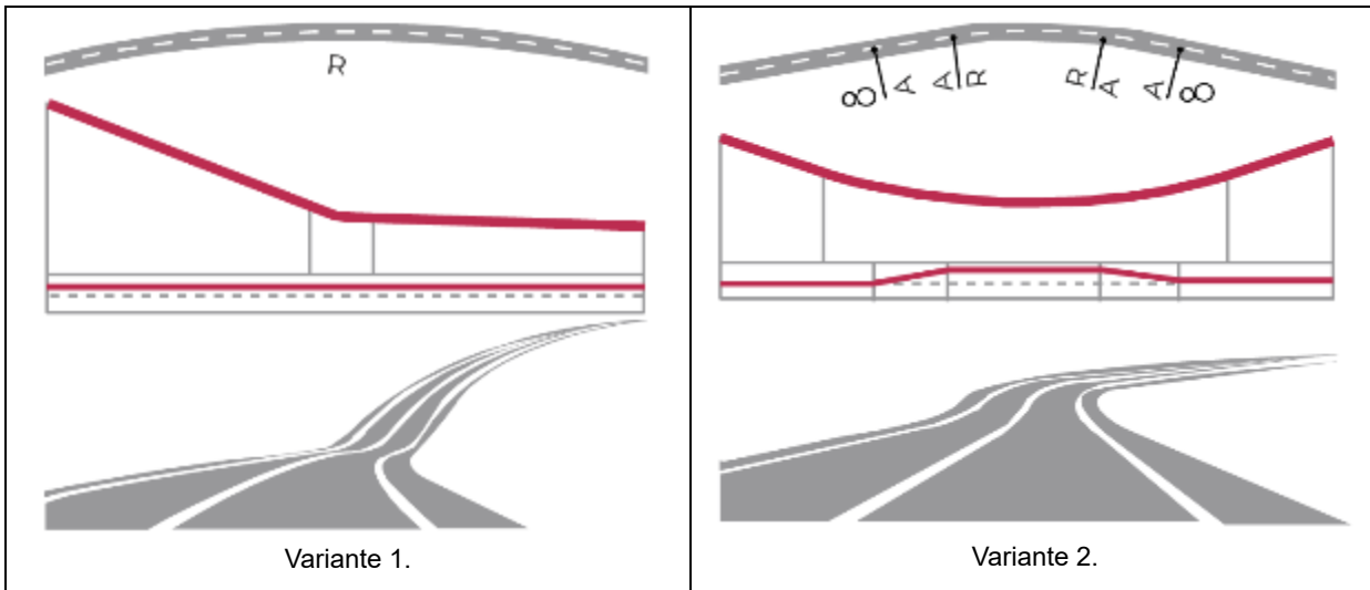
Figura 20.- Acentuada desproporción entre elementos de trazo [1] [2]
