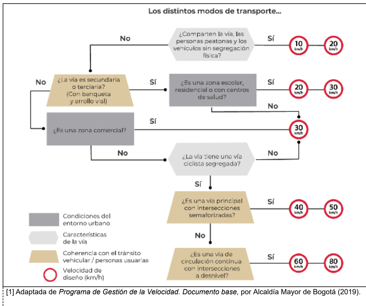
Figura 31.- Diagrama de flujo para establecer velocidades seguras [1]
