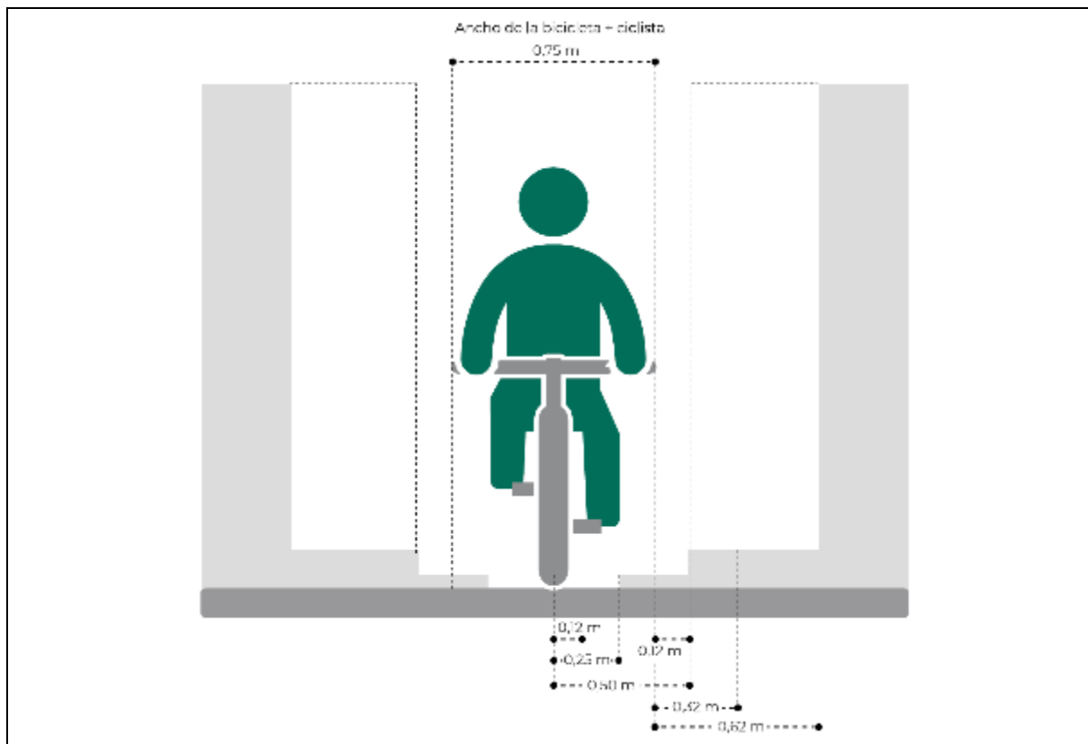
Figura 6.- Distancias de seguridad de las personas usuarias [1] [2]
