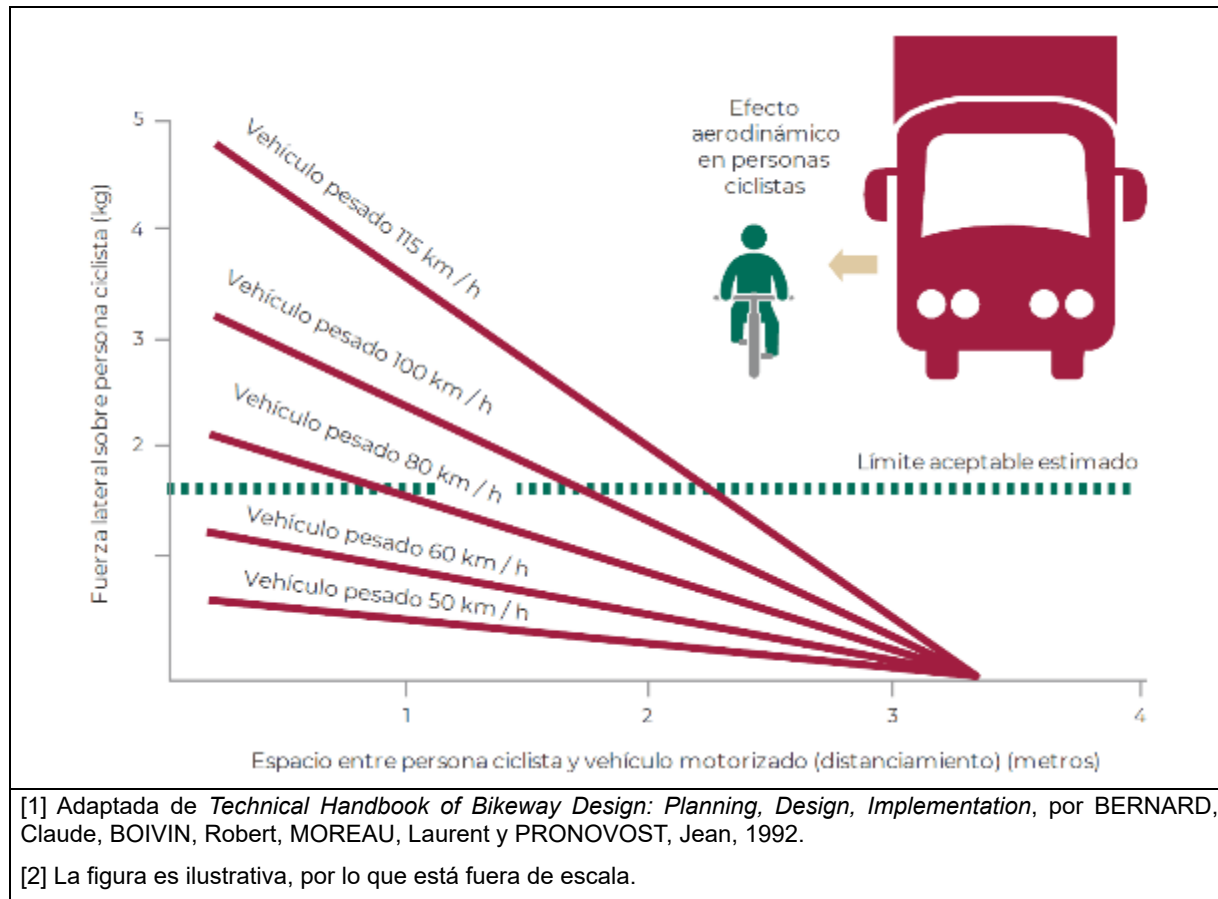
Figura 27.- Separación de vía ciclista debido al efecto aerodinámico [1] [2]
