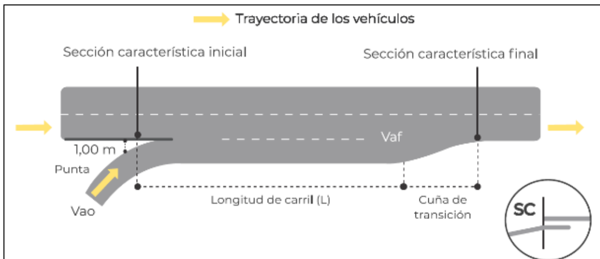
Figura 22.- Carriles de cambio de velocidad [1] [2] [a] [b]
