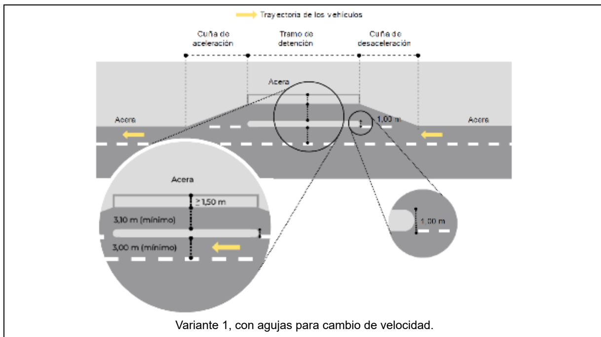
Figura 78.- Paradas de vehículos de transporte público de pasajeros [1] [2]
