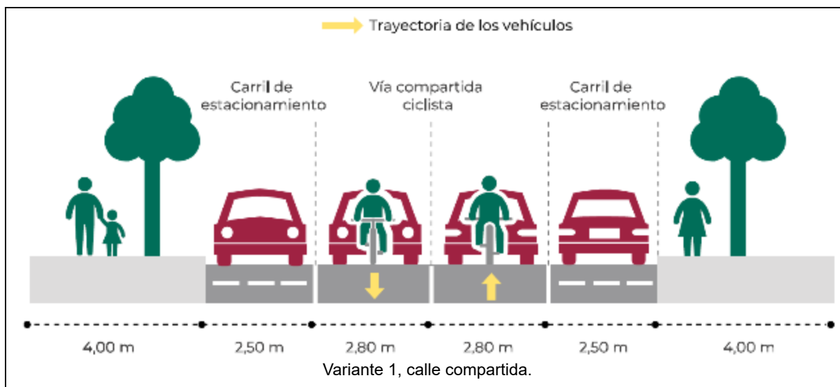
Figura 48.- Perfil tipo de vía ciclista con prioridad de uso [1] [2] [3]
