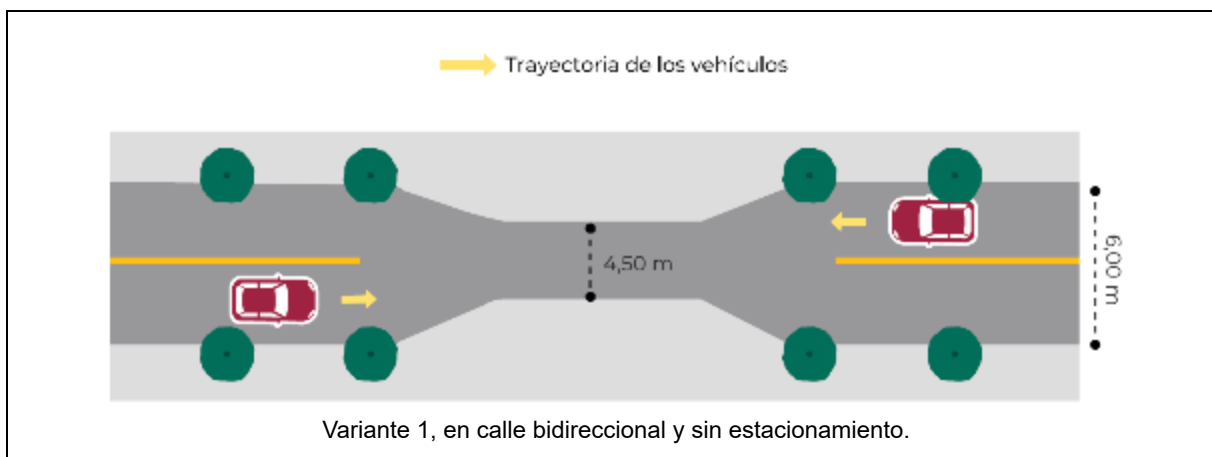
Figura 106.- Tipos de estrechamientos laterales [1] [2]
