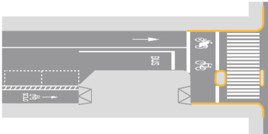
Variante 3, parada con plataforma a nivel de acera en cicloavía confinada por carril de estacionamiento.
