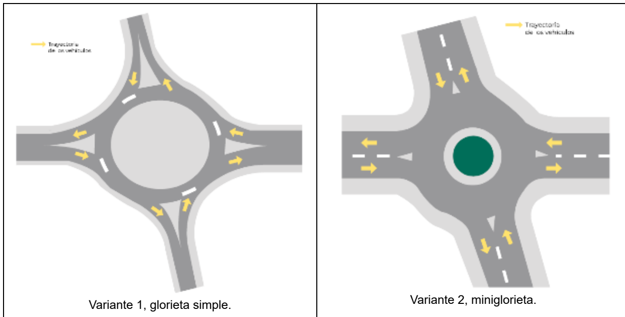
Figura 88.- Tipos de intersecciones giratorias [1] [2]
