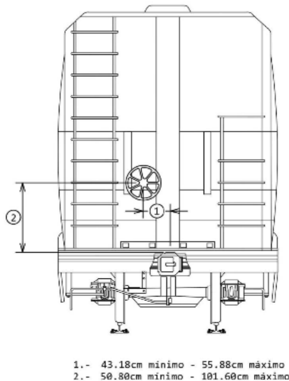
Fig. 8 Freno vertical. Localización de la flecha del freno.
