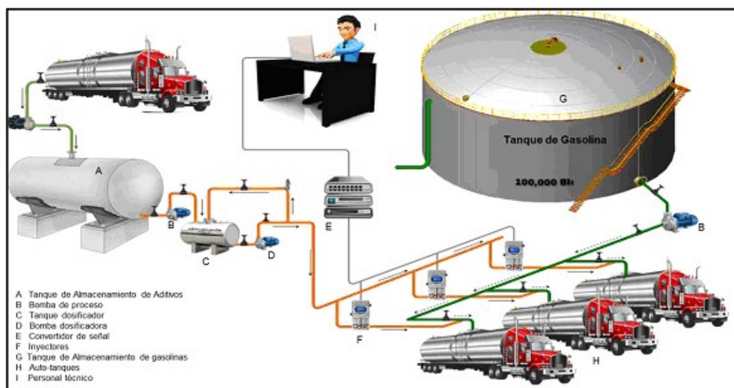
Figura 7. Sistema automático de dosificación de Aditivos
