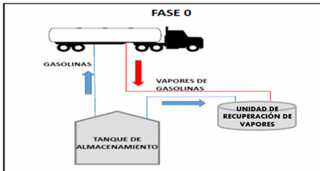
Figura 6. Fase 0 del Sistema de Recuperación de Vapores
