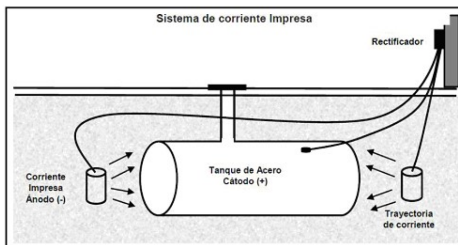
Figura 2. Sistema de protección catódica por corriente impresa
