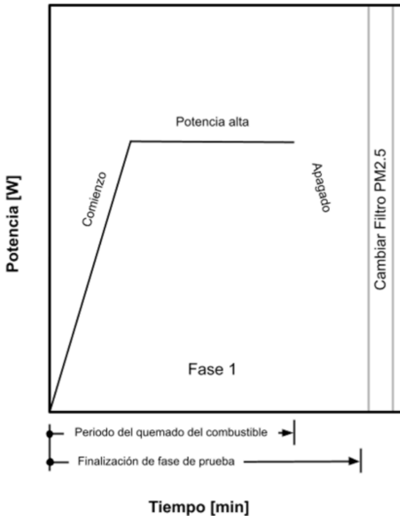
Figura 1 - Diagrama de la secuencia de la prueba estándar para estufas con un solo nivel de potencia En la Figura 2 se ilustra la secuencia de la prueba estándar para estufas con un rango de potencia de cocción.
