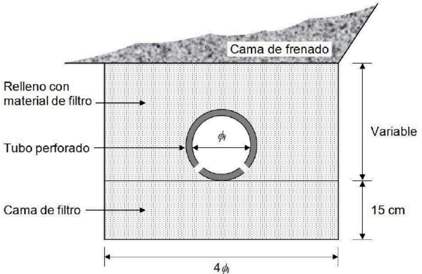
FIGURA 5.- Subdrén típico para la cama de frenado
