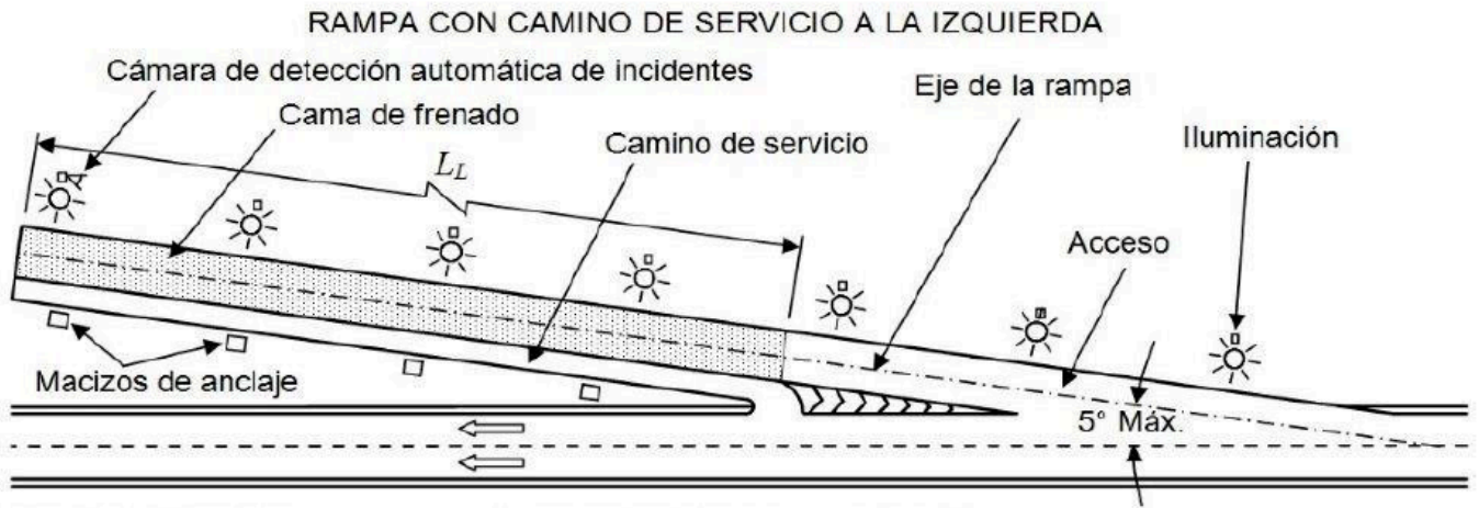
FIGURA 1.- Rampa de emergencia para frenado. Esquema de disposición en planta
