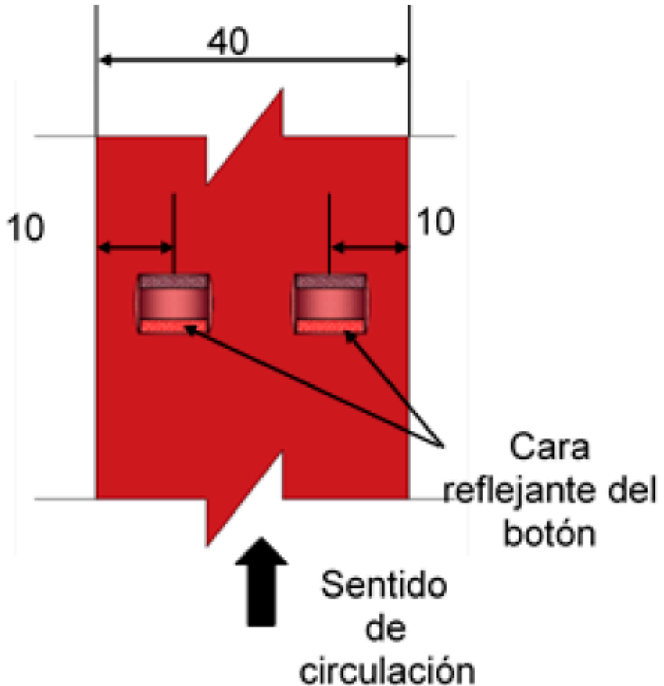
FIGURA 7.- Ubicación de los botones reflejantes
