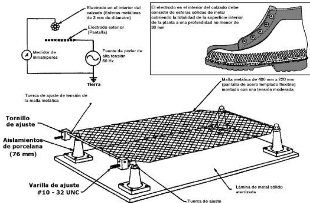
Figura 5. Ejemplo del aparato de prueba para rigidez dieléctrica
