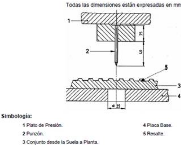
Figura 12. Aparato para la prueba de resistencia a la penetración
