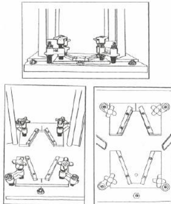
Figura 9. Ejemplo de dispositivo de sujeción para calzado con protección metatarsal
