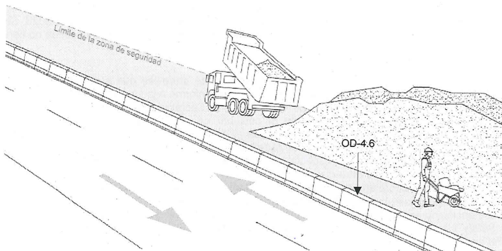
FIGURA 25.- Barrera en zona de obra (OD-4.6)
