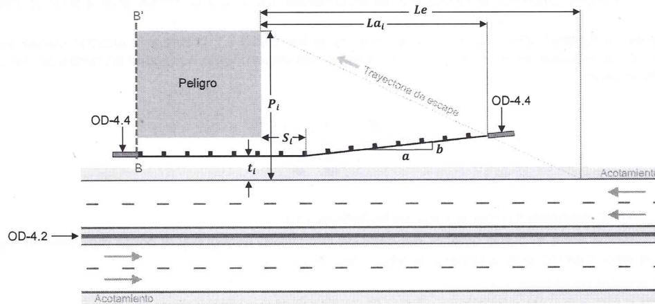
FIGURA 13.- Instalación de barrera de orilla de corona (OD-4.1) en carretera con sentidos de circulación separados
