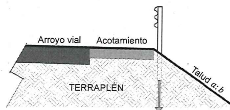
b) Barrera de orilla de corona instalada sobre talud de terraplén
