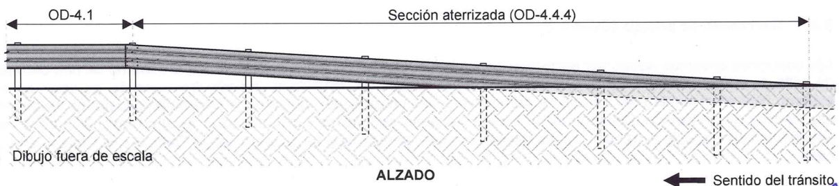
FIGURA 24.- Sección aterrizada para vigas acanaladas (OD-4.4.4)
