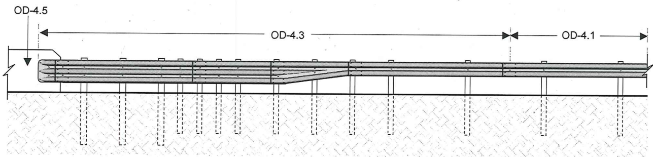
FIGURA 20.- Sección de transición (OD-4.3) conectando una barrera de orilla de corona (OD-4.1) a un parapeto para vehículo motorizado (OD-4.5)
