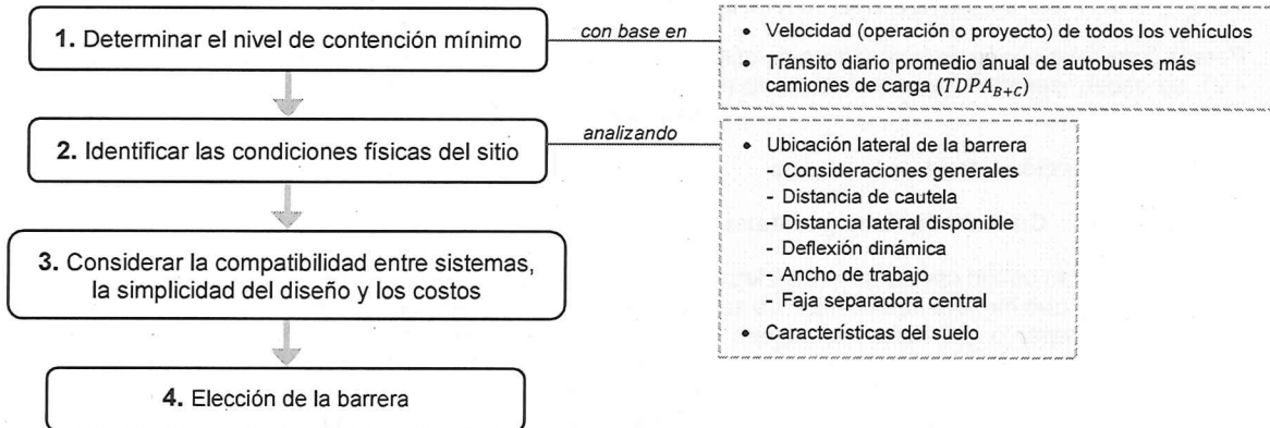
FIGURA 4. Proceso para seleccionar una barrera de orilla de corona (OD-4.1) o separadora de sentidos de circulación (OD-4.2)
