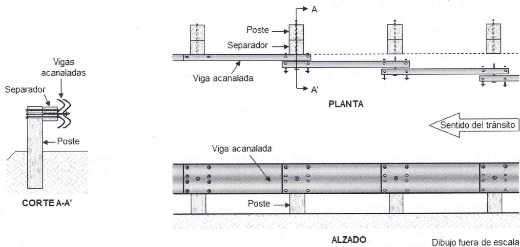
FIGURA 19.- Instalación de vigas acanaladas de acero
