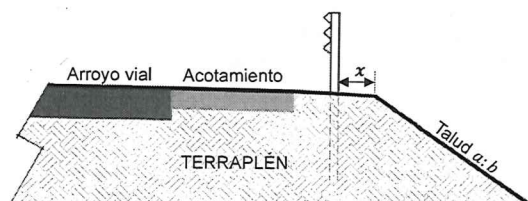
a) Barrera de orilla de corona instalada sobre la corona
